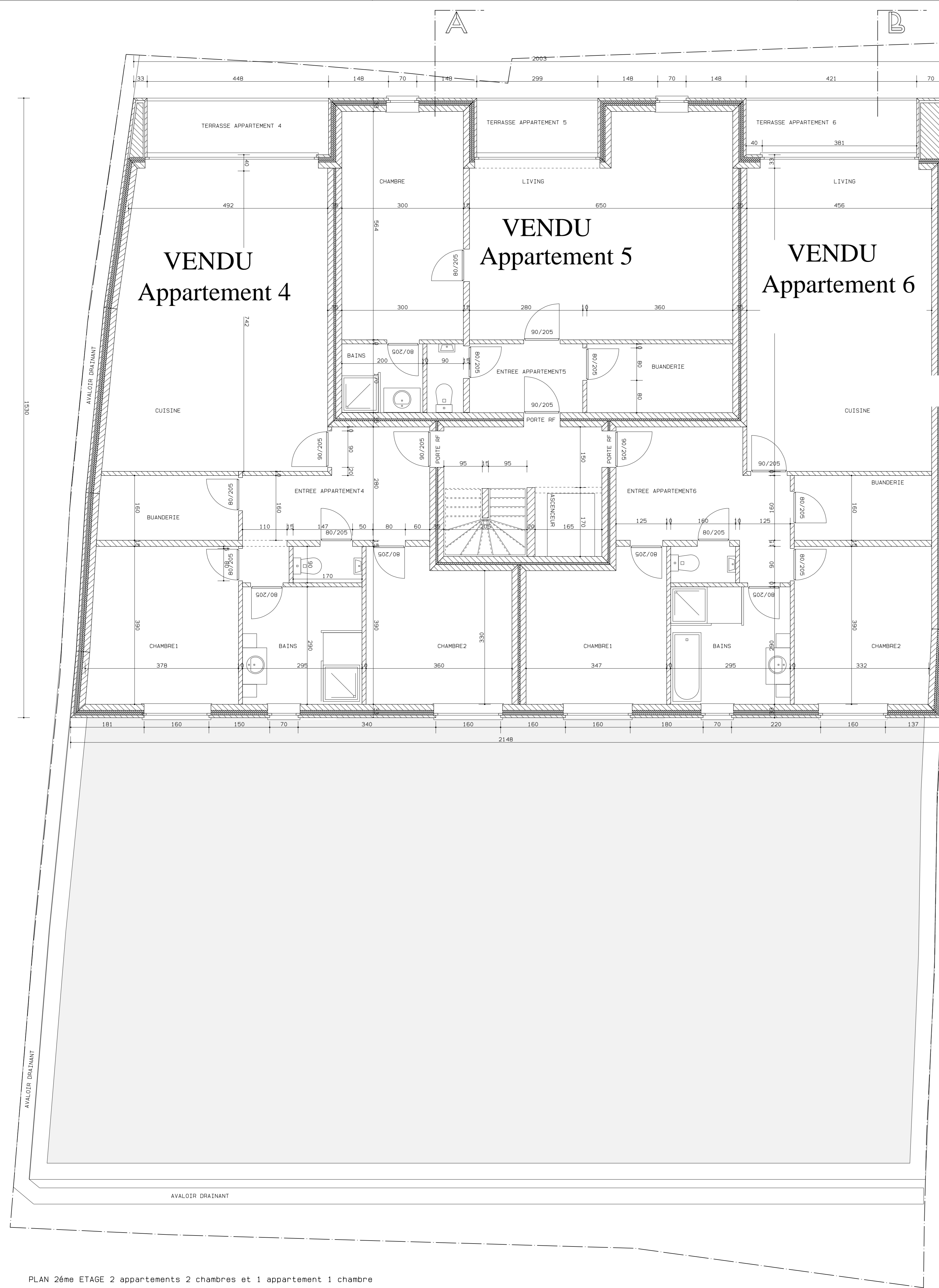
PLAN 26 me ETAGE 2 appartements 2 chambres et 1 appartement 1 chambre APPARTEMENTS 4/5/6
