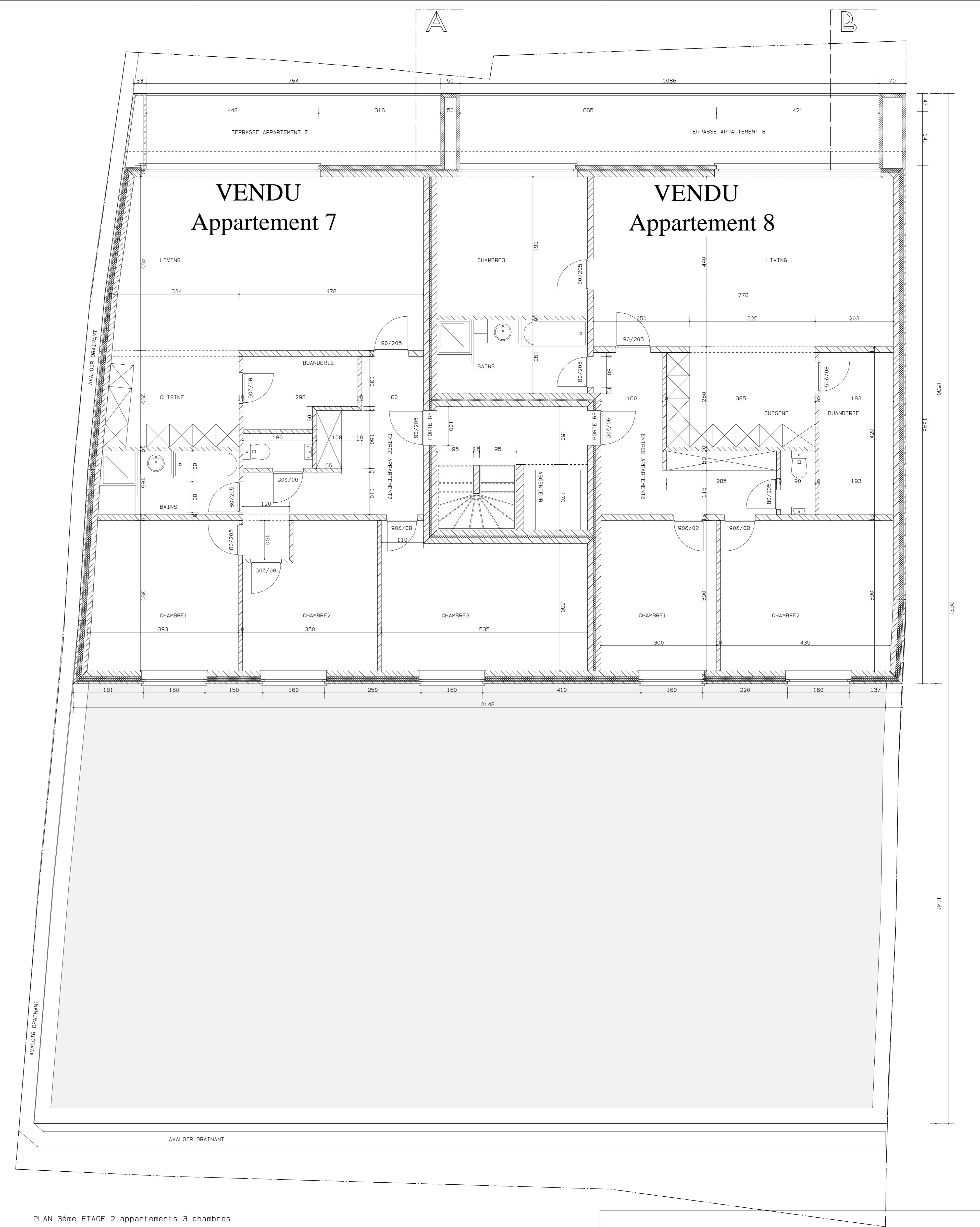
PLAN 36 me ETAGE 2 appartements 3 chambres APPARTEMENTS 7/8/9
